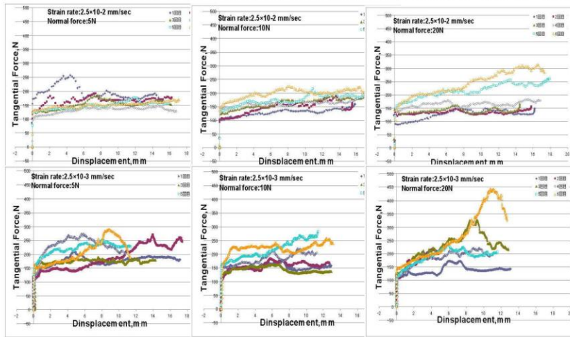
岩手大学吉野准教授の下測定した Test piece 10mm×60mm×t10mm S45CとSKD61での横滑り試験データ (全てn=6)
